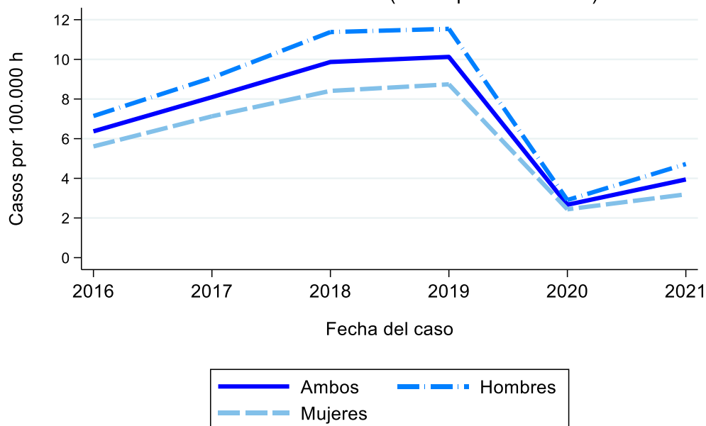
Figura 1. Vigilancia de Giardiasis. 2016-2021 Incidencia acumulada (casos por 100.000 h.)
