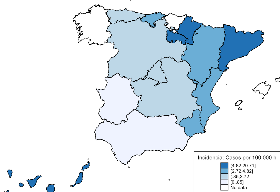
Figura 2. Vigilancia de Giardiasis. España. 2021 Incidencia acumulada por Comunidades Autónomas
