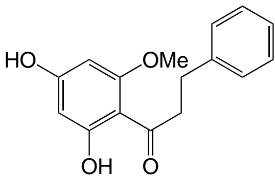
Cardamonin
