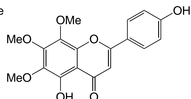
Xanthomicrol
