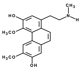
#2 Secoboldine
