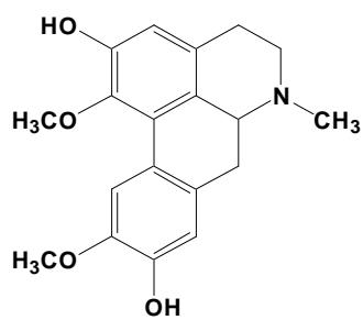
Boldine
