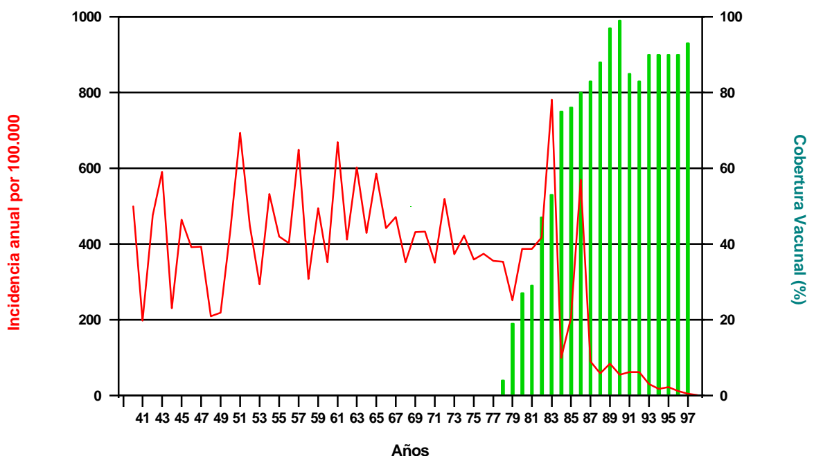
Gráfica 1: Sarampión. España 1940-1998 Incidencia anual y cobertura de vacunación
