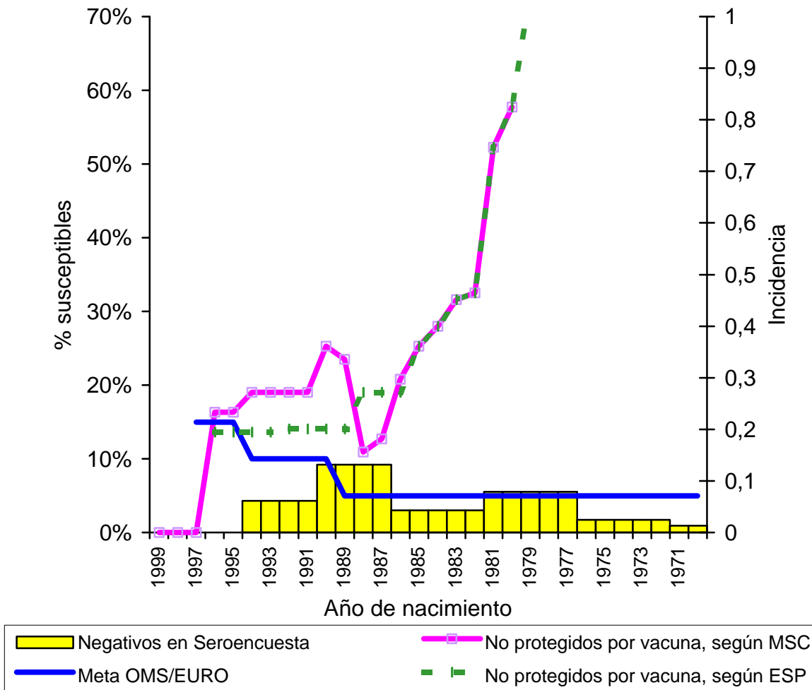
Gráfica 4: Estimación de la susceptibilidad a partir de datos de sarampión
