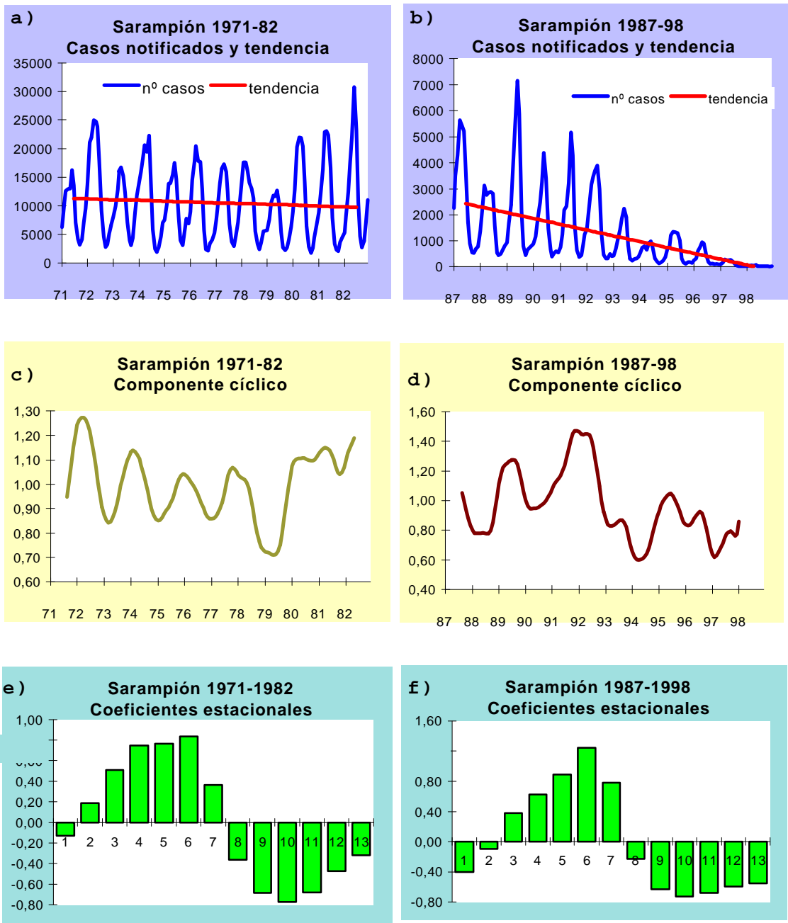
Gráfica 2: Series temporales de sarampión
