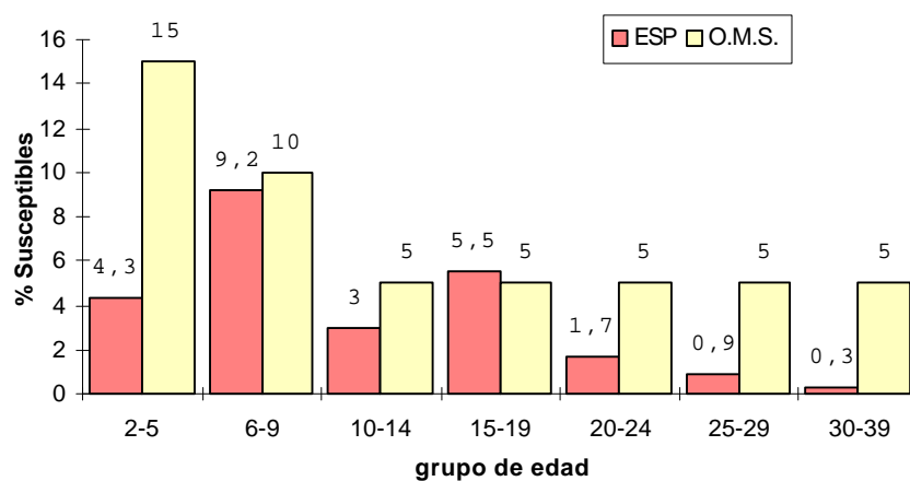
Gráfica 3: Sarampión, población susceptible por edad
