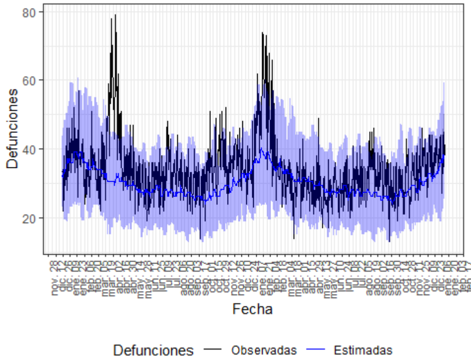
Figura 12. Mortalidad por todas las causas observada y esperada. Extremadura, diciembre 2019 hasta 11 de enero de 2022.
