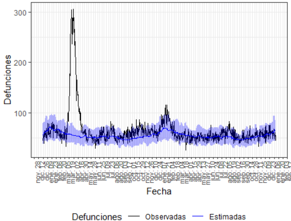
Figura 9. Mortalidad por todas las causas observada y esperada. Castilla La Mancha, diciembre 2019 hasta 11 de enero de 2022.
