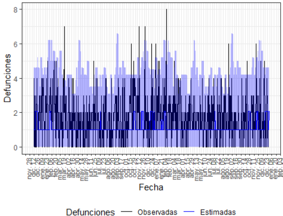
Figura 19. Mortalidad por todas las causas observada y esperada. Ceuta, diciembre 2019 hasta 11 de enero de 2022.
