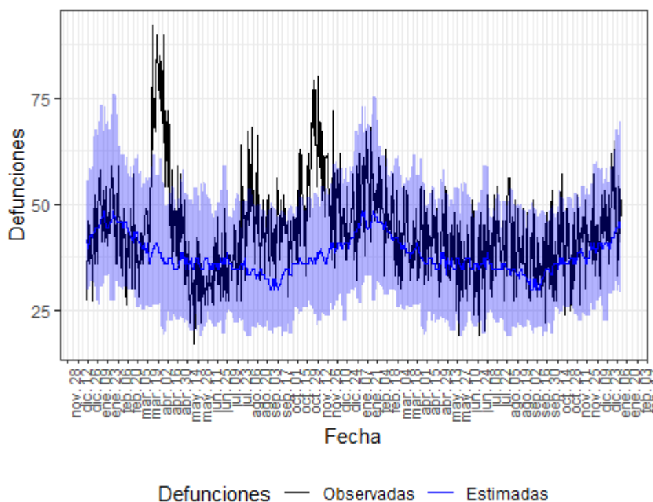
Figura 3. Mortalidad por todas las causas observada y esperada. Aragón, diciembre 2019 hasta 11 de enero de 2022.
