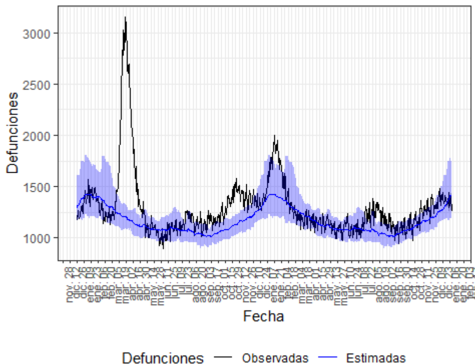
Figura 1. Mortalidad por todas las causas observada y esperada. España, diciembre 2019 hasta 11 de enero de 2022
