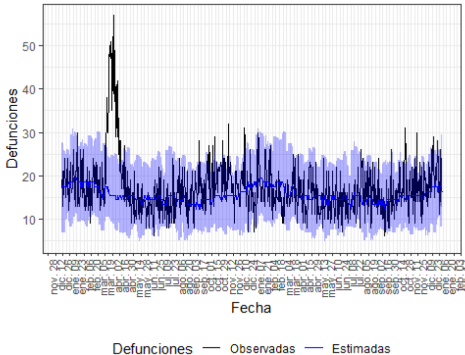
Figura 16. Mortalidad por todas las causas observada y esperada. Navarra, diciembre 2019 hasta 11 de enero de 2022.
