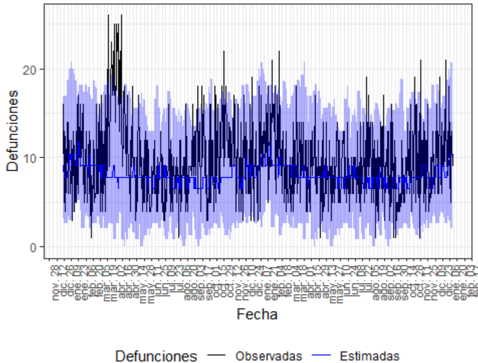
Figura 18. Mortalidad por todas las causas observada y esperada. La Rioja, diciembre 2019 hasta 11 de enero de 2022.
