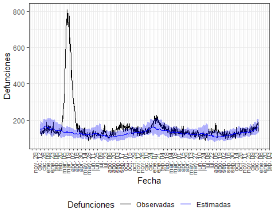
Figura 14. Mortalidad por todas las causas observada y esperada. Comunidad de Madrid, diciembre 2019 hasta 11 de enero de 2022.
