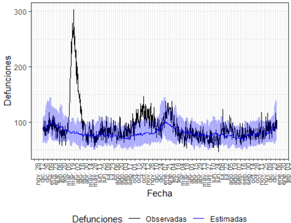
Figura 8. Mortalidad por todas las causas observada y esperada. Castilla y León, diciembre 2019 hasta 11 de enero de 2022.
