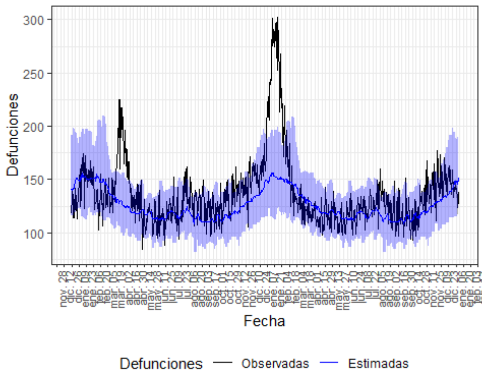
Figura 11. Mortalidad por todas las causas observada y esperada. Comunitat Valenciana, diciembre 2019 hasta 11 de enero de 2022.
