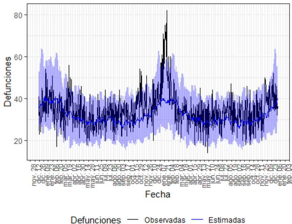
Figura 15. Mortalidad por todas las causas observada y esperada. Murcia, diciembre 2019 hasta 11 de enero de 2022.
