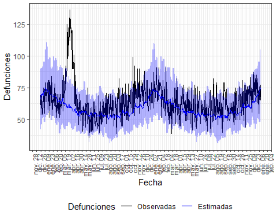
Figura 17. Mortalidad por todas las causas observada y esperada. País Vasco, diciembre 2019 hasta 11 de enero de 2022.
