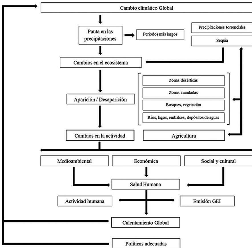
Figura 1: Visión esquemática de la problemática del cambio climático
